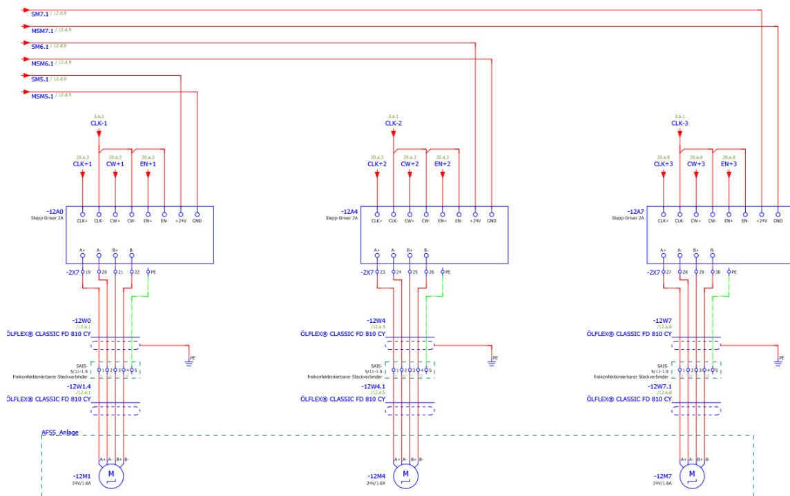
Abbildung 4.11: 40Ncm Schrittmotoren im Schaltplan
