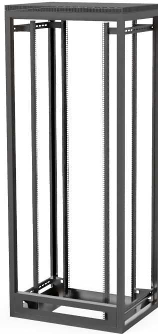
Abbildung 4.5: Serverschrank konstruiert
