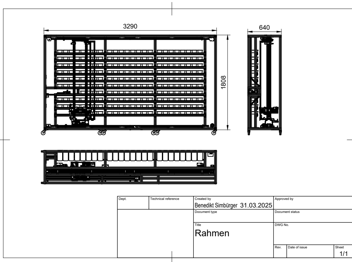
Abbildung 7.1: Abmessungen Rahmen
