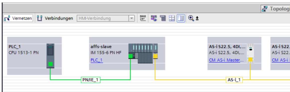
Abbildung 5.9: Netzsicht im TIA-Portal mit ASi-Master und Slaves
