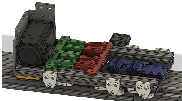
(a) X-Schuttle Ansicht hinten (Motor rechts und Rollen ausgeblendet)
