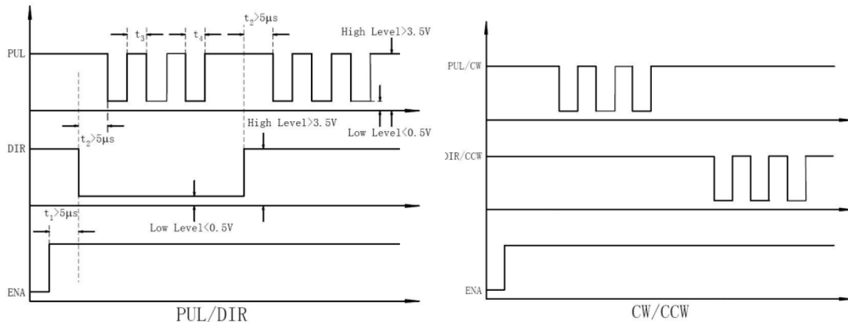
Abbildung 3.4: Sequenzdiagramm der Kontrollsignale, Quelle: [33]
