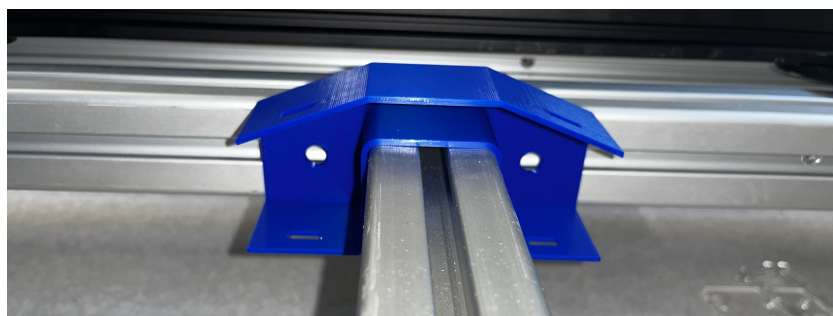
Abbildung 5.11: Kabelbrücke x-Achse
