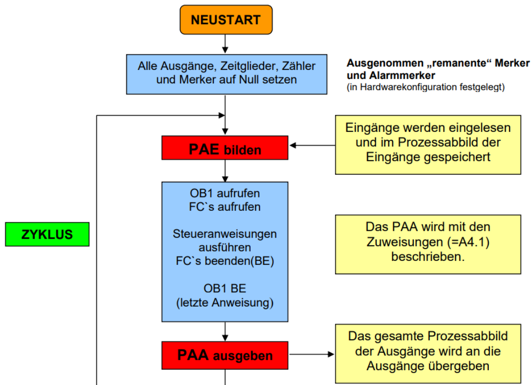
Abbildung 3.1: Arbeitsweise einer SPS, Quelle: [26]
