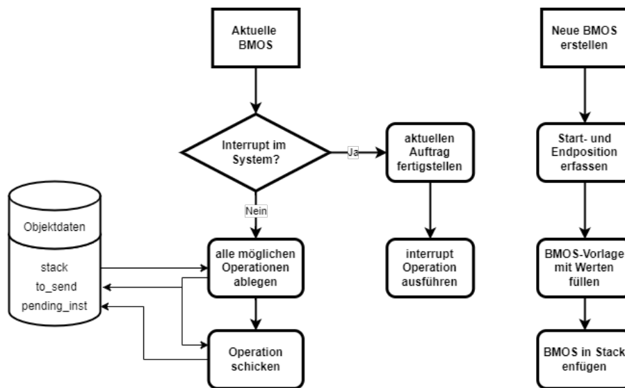
Abbildung 2.14: Diagramm der BMOS bereitstellung
