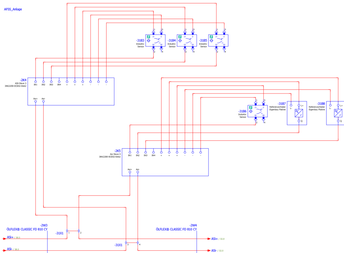
Abbildung 4.12: Sensoren mit den ASi-Slaves, erste Seite von vier
