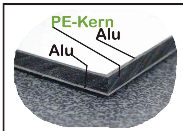
Abbildung 4.2: Dibond-Platte, Quelle: [40]
