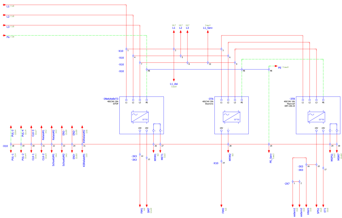
Abbildung 4.8: Schaltplan: Netzteile
