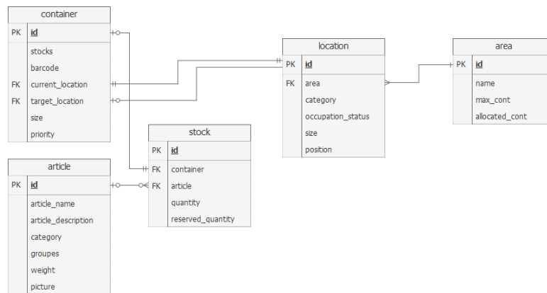
Abbildung 2.15: Datenbankschema des AFSS
