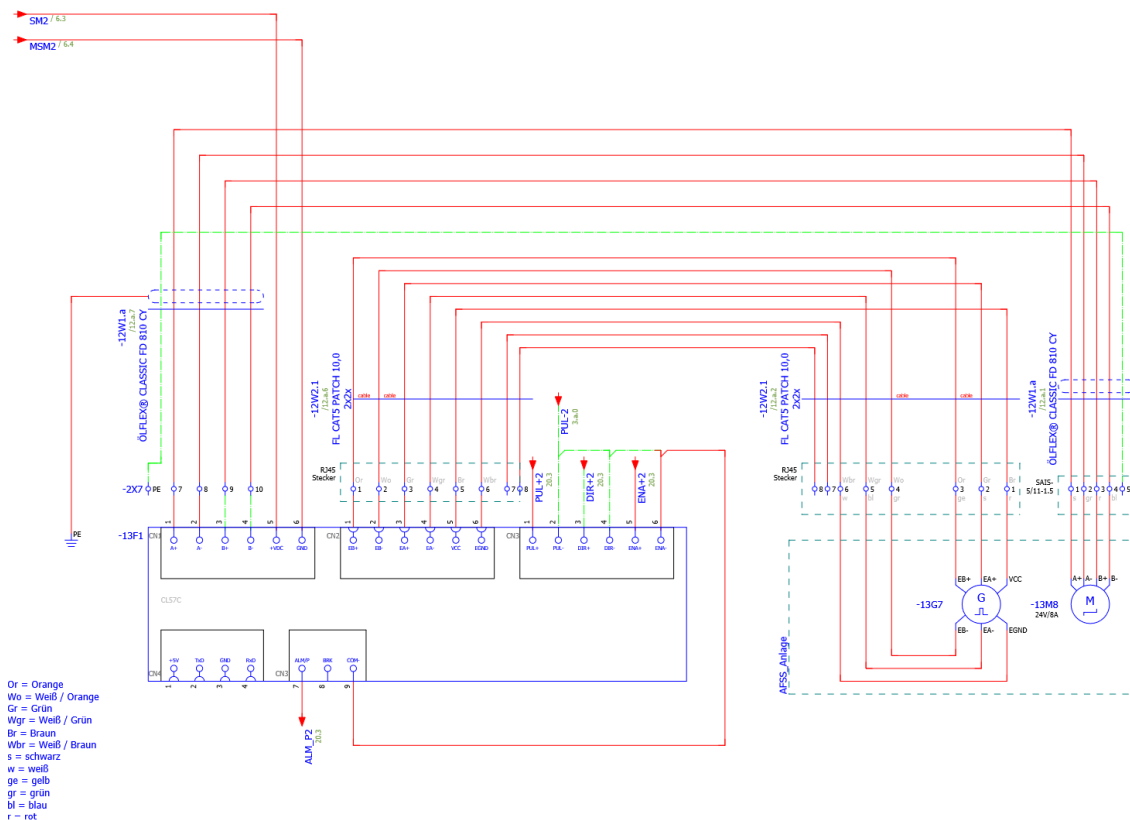
Abbildung 4.9: Seite 13 des Schaltplans, SM ohne Bremse
