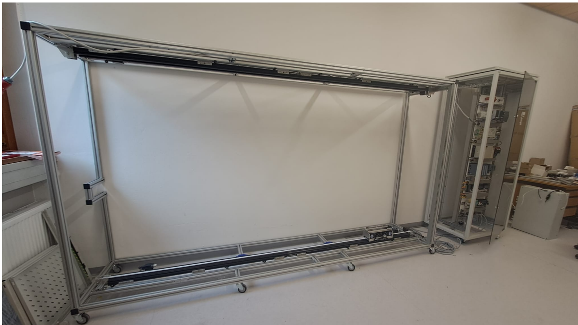
Abbildung 2.11: Aufgebauter Rahmen und X-Achse
