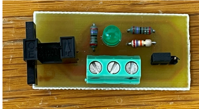
Abbildung 5.4: Fertige Referenzplatine
