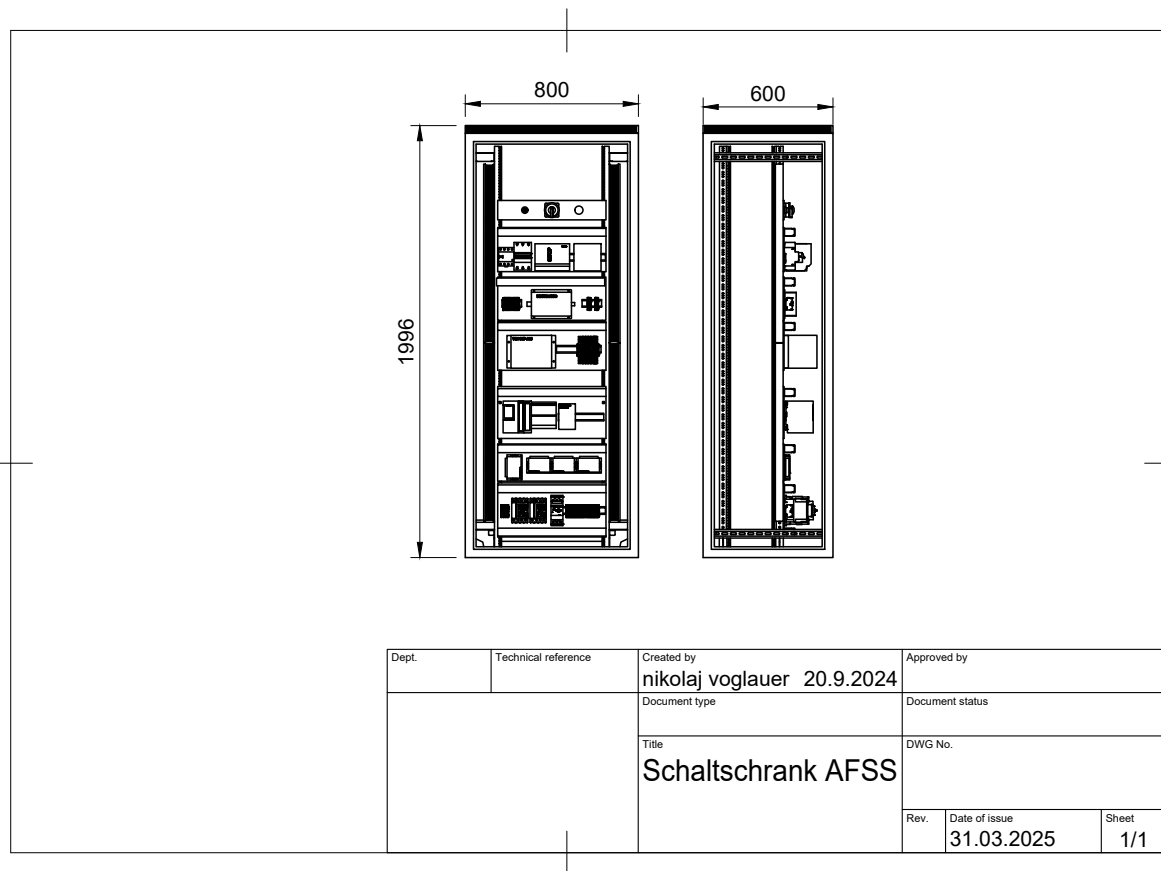
Abbildung 7.2: Abmessungen Schaltschrank
