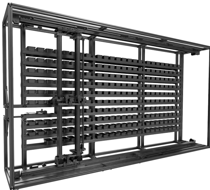
Abbildung 2.12: Gesamtkonstruktion
