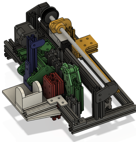
(a) YZ-Achse, zweite Hälfte ausgeblendet
