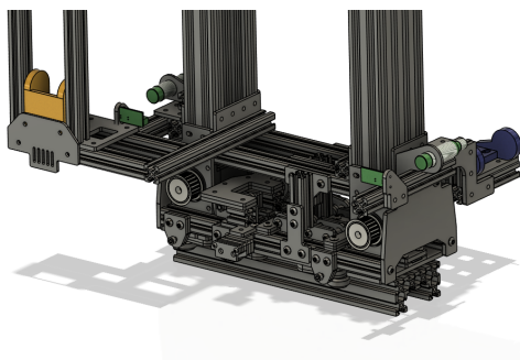
(a) X-Schuttle unten mit Anbauten
