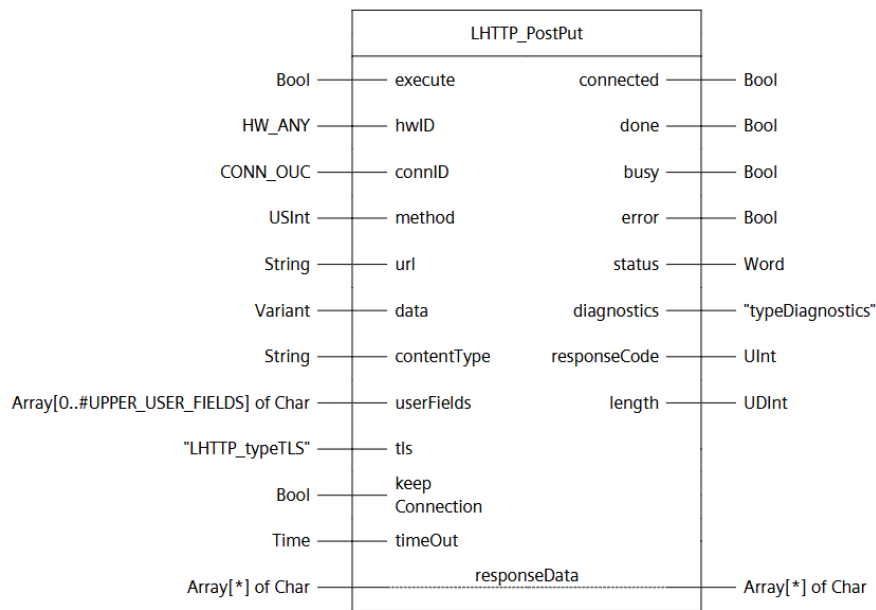
Abbildung 3.7: POST-Put Baustein, Quelle: [38]
