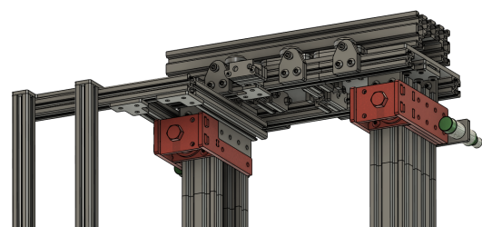
(b) X-Shuttel oben
