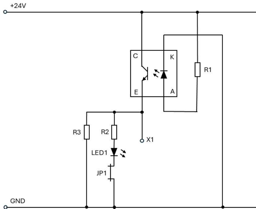
Abbildung 5.2: Schaltplan Referenzplatine
