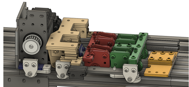
(b) X-Schuttle Ansicht vorne (Motor rechts und Profil vorne ausgeblendet)
