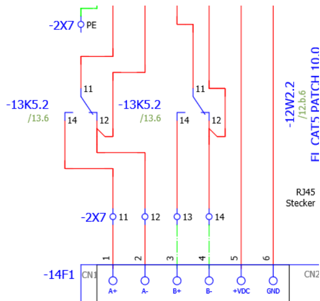
Abbildung 4.10: Zusätzliche Kurzschließung von Spulen bei horizontalen Antrieben
