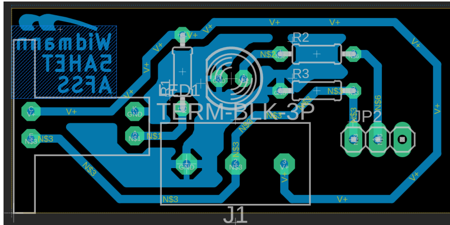
Abbildung 5.3: Leiterplattenplan Referenzplatine
