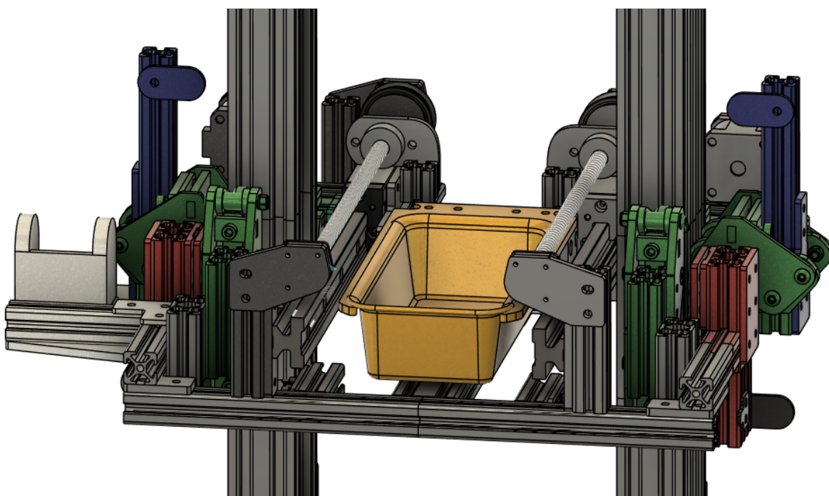
Abbildung 2.8: XY-Shuttel Gesamtansicht
