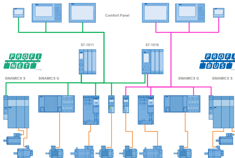
Abbildung 5.8: Topologie verschiedener Feldbussysteme, Quelle: [61]
