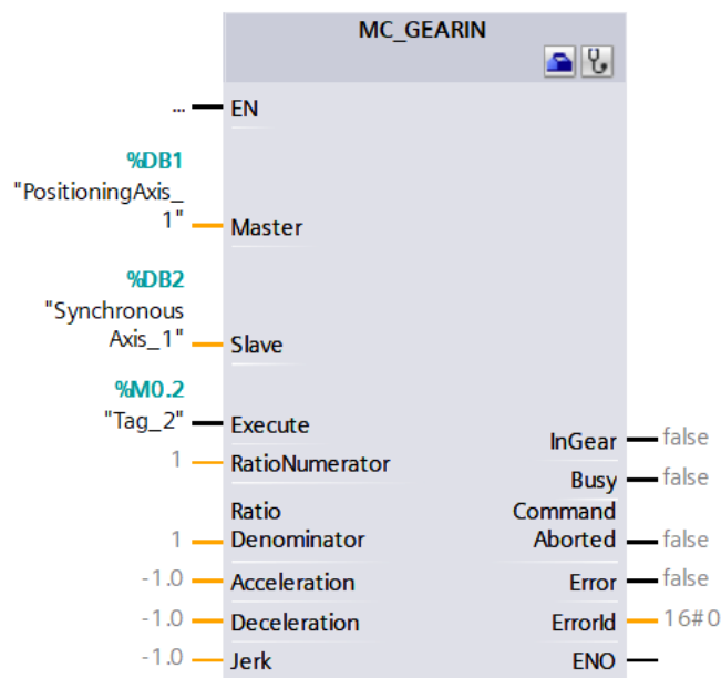
Abbildung 3.5: Baustein MC_GearIn
